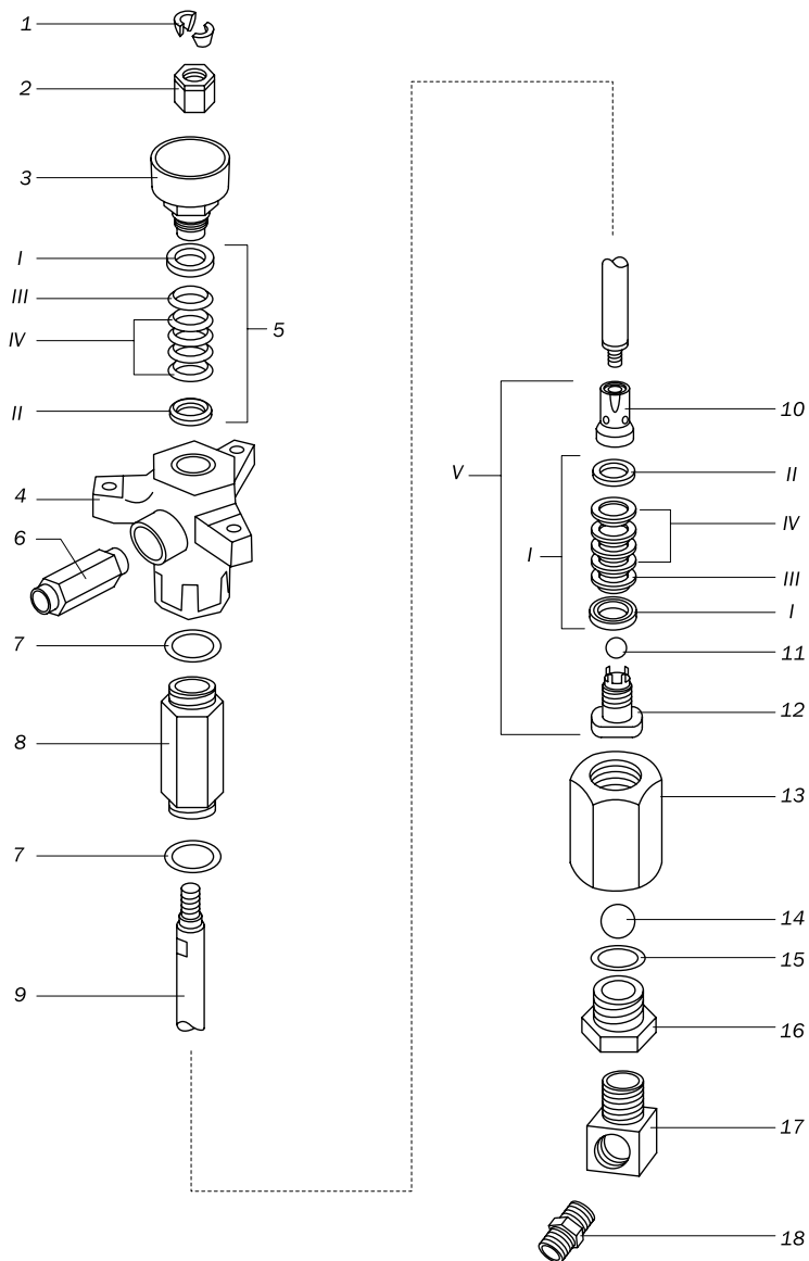
Рис. 9.2.1. Деталировочный чертеж насоса окрасочного аппарата.
