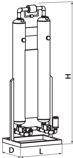
рис. 1 Габаритная схема осушителя AD
